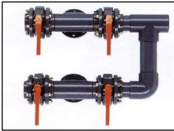
BATERIA 4 VALVULAS MANUAL O AUTOMATICA
