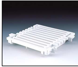
REJILLA TRANSVERSAL UNION ENGANCHES A PRESION Largo: 19'5 cm Ancho 245 Cod. 00217 Ancho 295 Cod. 00218 Ancho 335 Cod. 00219
